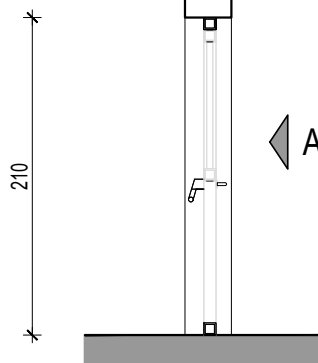
PRESEK 1-1
