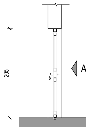
PRESEK 1-1
