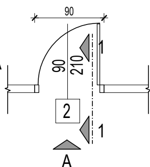
OSNOVA
