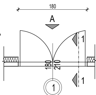
OSNOVA
