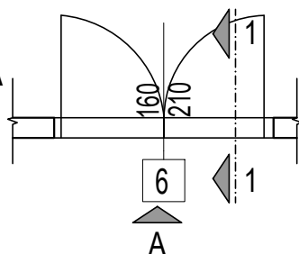
OSNOVA
