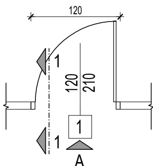
OSNOVA
